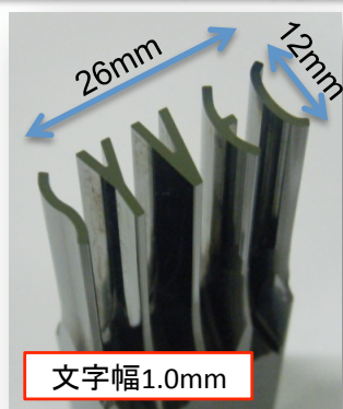
写真2 鏡面SYVECパンチ
