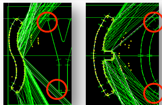
図1 シミュレーションによる干渉チェック
